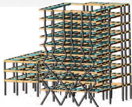
おおたかの森3D CAD図面
