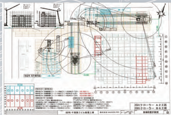
重機配置計画図
